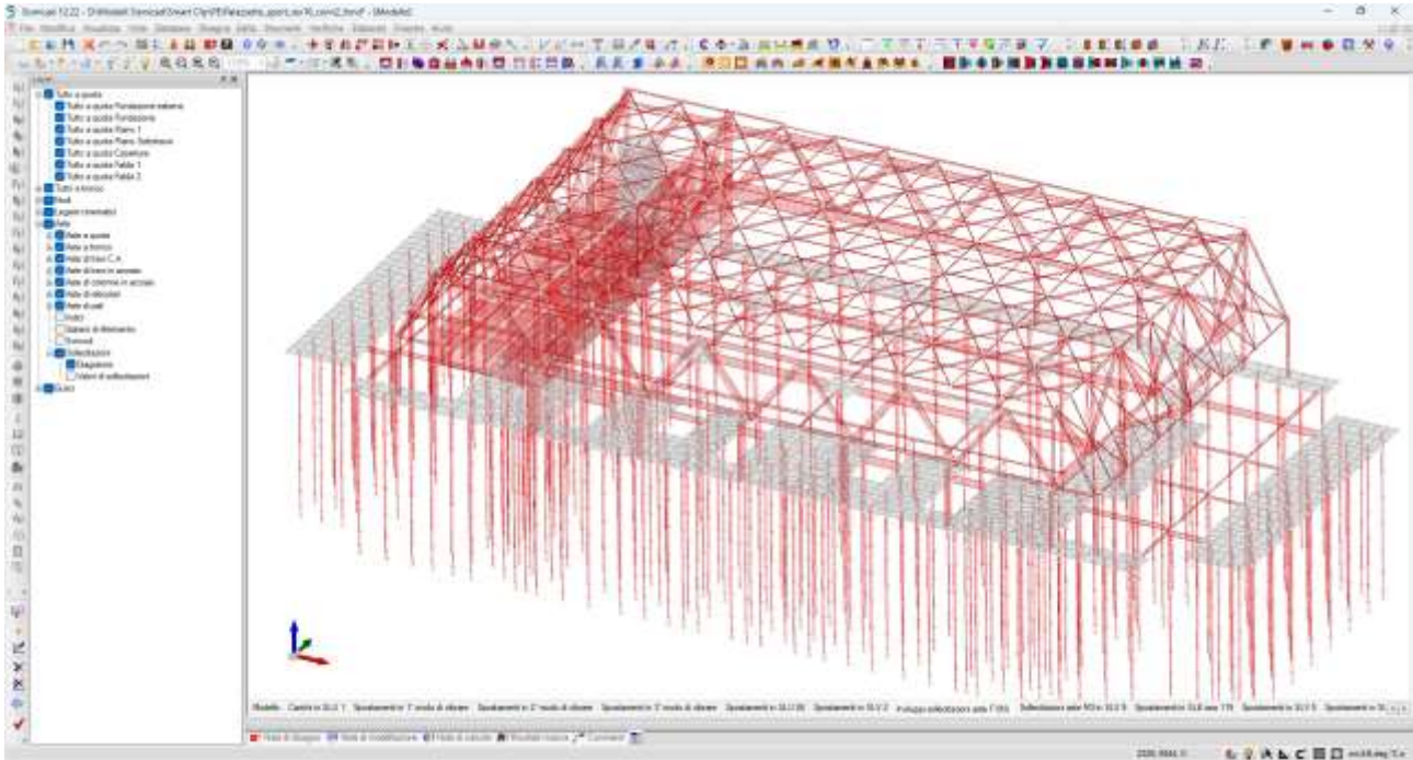
Figura 8. Involuppo sforzo normale SLU/SLV
