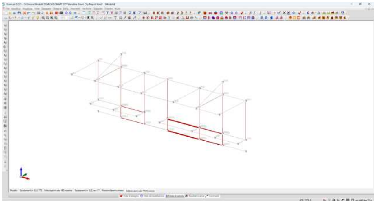
Figura 20. Involuppo sforzo normale SLU/SLV
