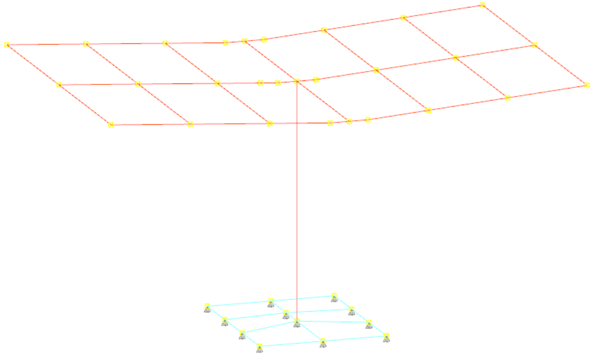
Figura 6. Modello analitico Stazionamento
