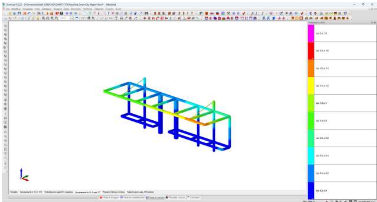
Figura 25. Spostamenti in esercizi
