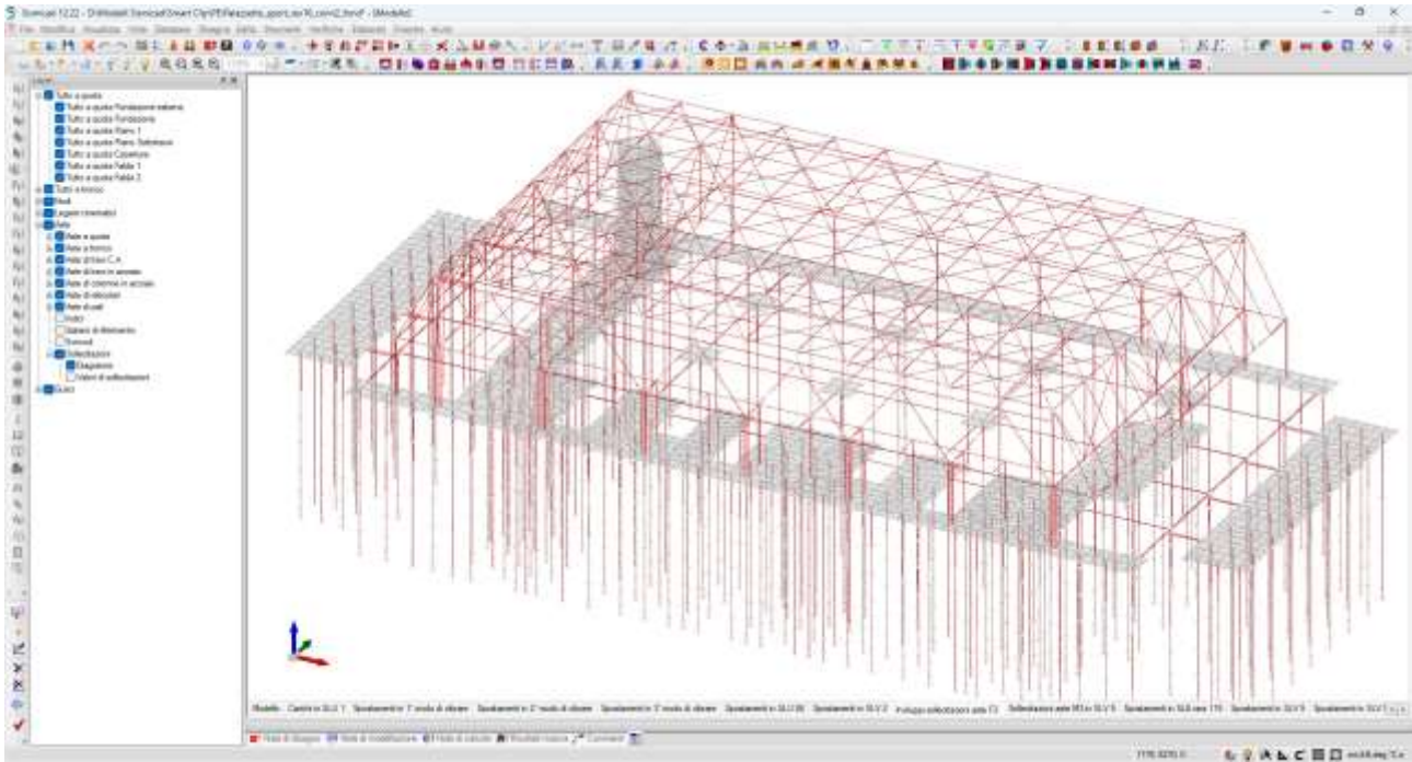
Figura 10. Involuppo taglio F3 SLU/SLV
