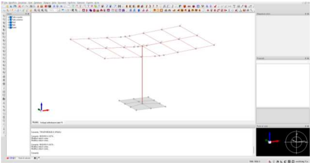
Figura 16. Involuppo taglio F3 SLU/SLV
