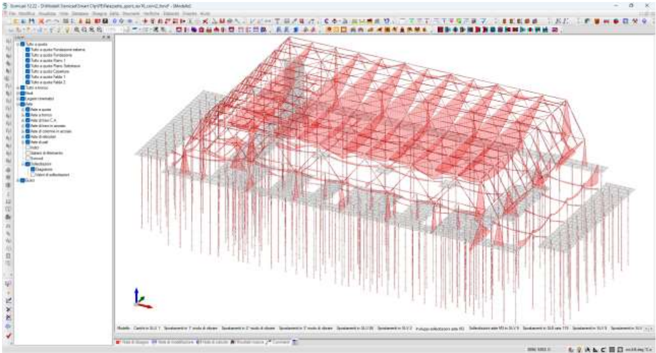
Figura 12. Involuppo momento M3 SLU/SLV
