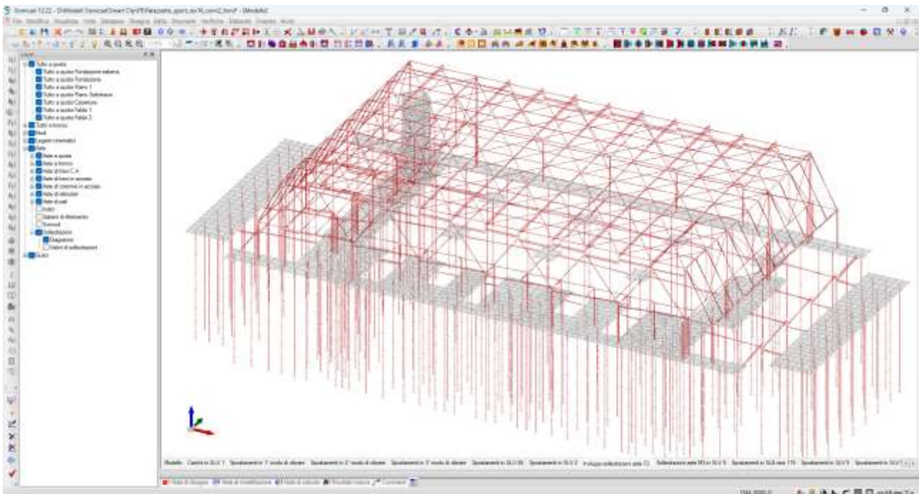
Figura 9. Involuppo taglio F2 SLU/SLV
