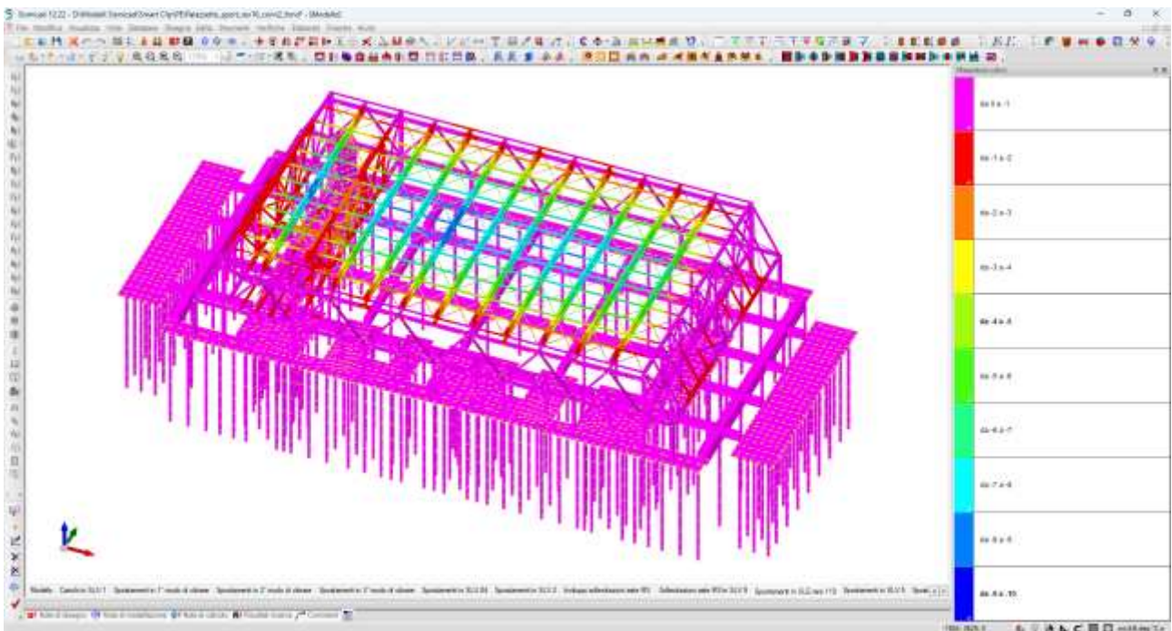
Figura 13. Spostamenti in esercizio
