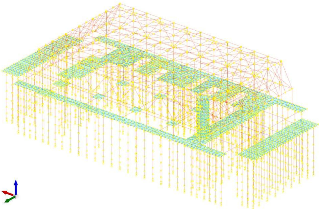
Figura 5. Modello analitico Palazzetto dello Sport
