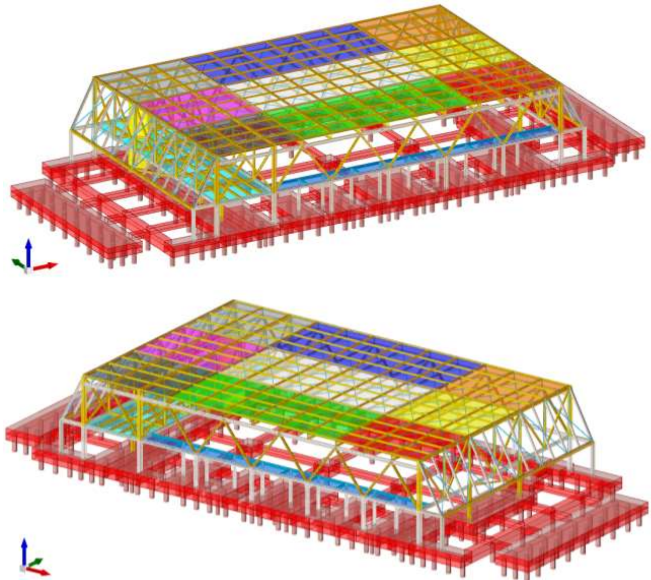
Figura 2. Viste 3D del modello geometrico Palazzetto dello Sport
